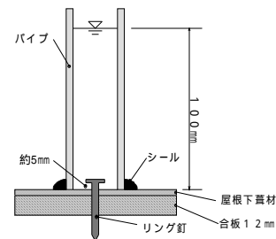
図1 釘穴周りの止水性試験
